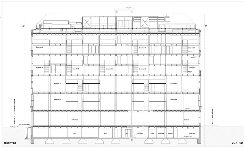
Schnitt B-B
