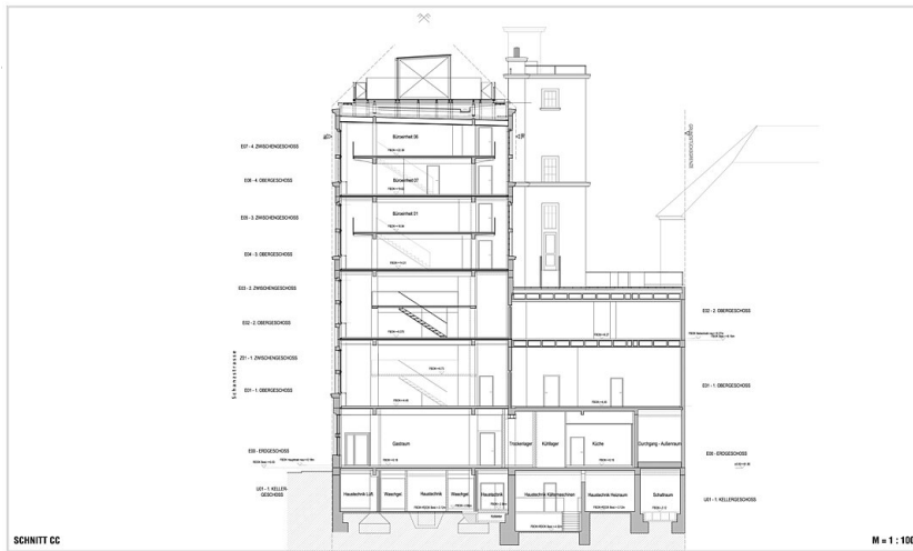
Schnitt C-C
