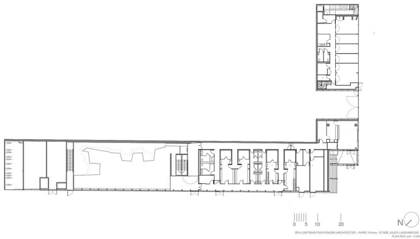
Grundriss EG
