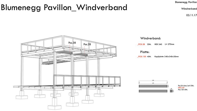
Perspektive Windverband
