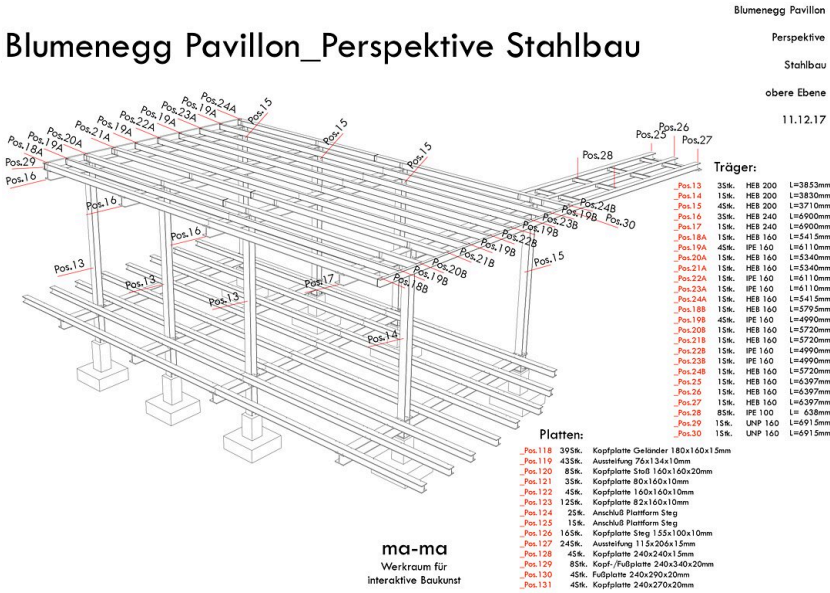
Perspektive Stahlbau
