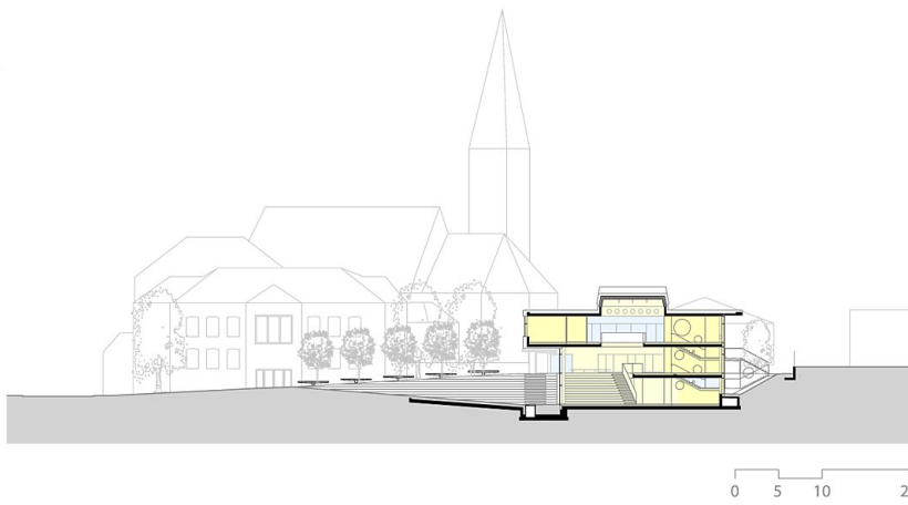
Querschnitt
