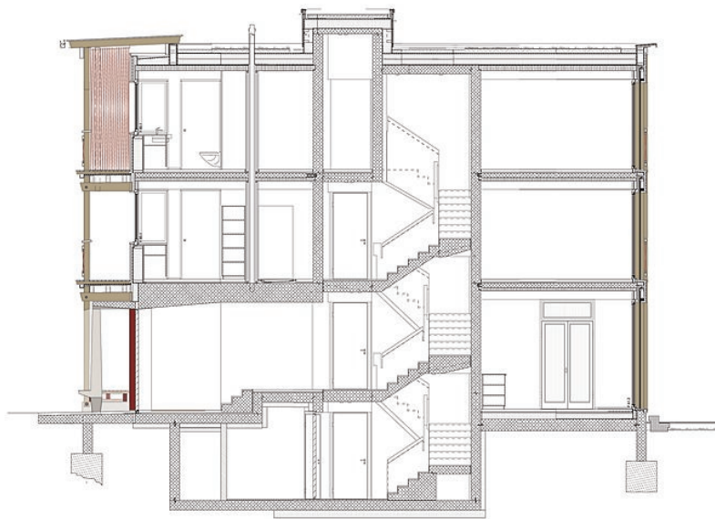
Fassadenschnitte S-Haus
