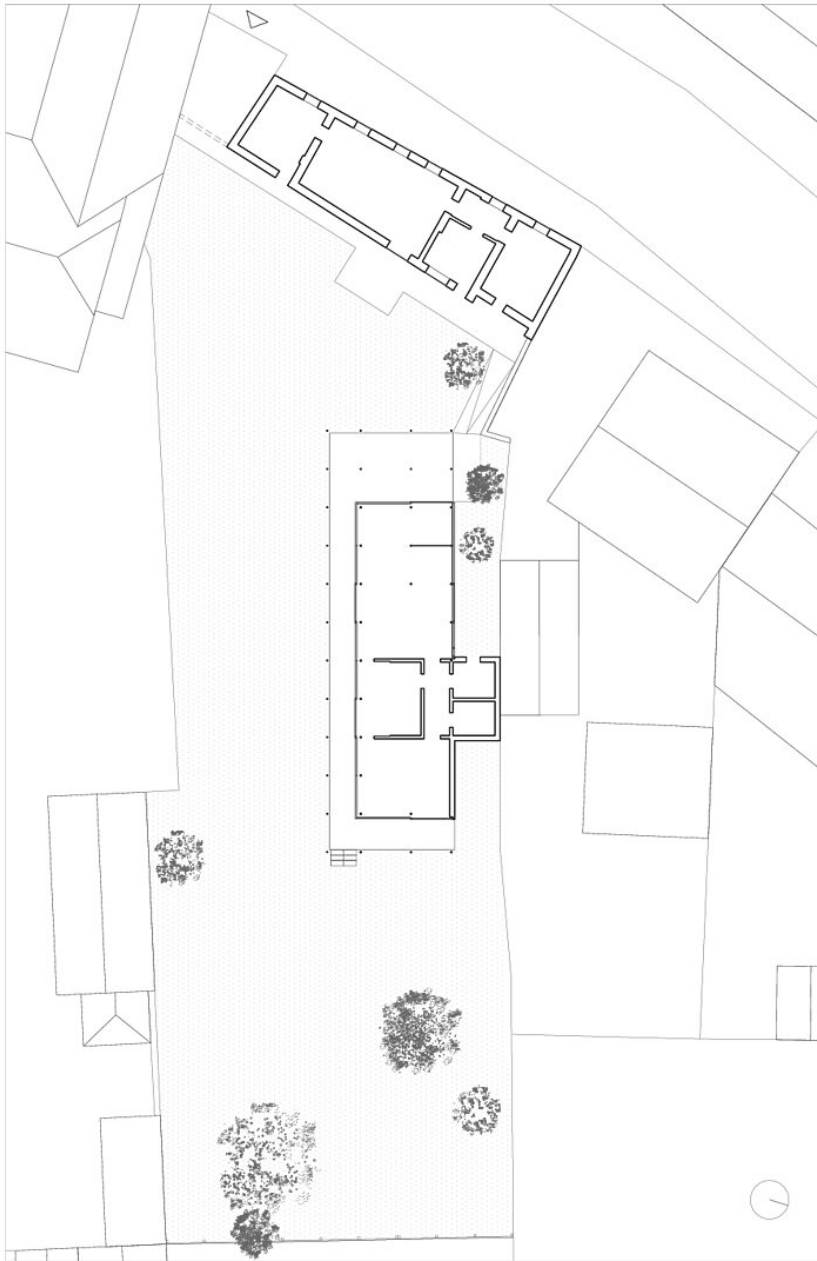
Lageplan
