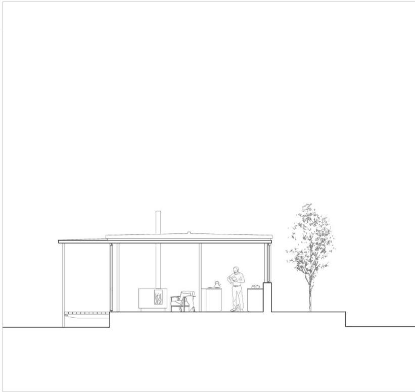
Schnitt AA
