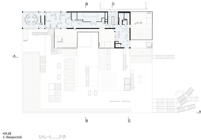
Grundriss OG5
