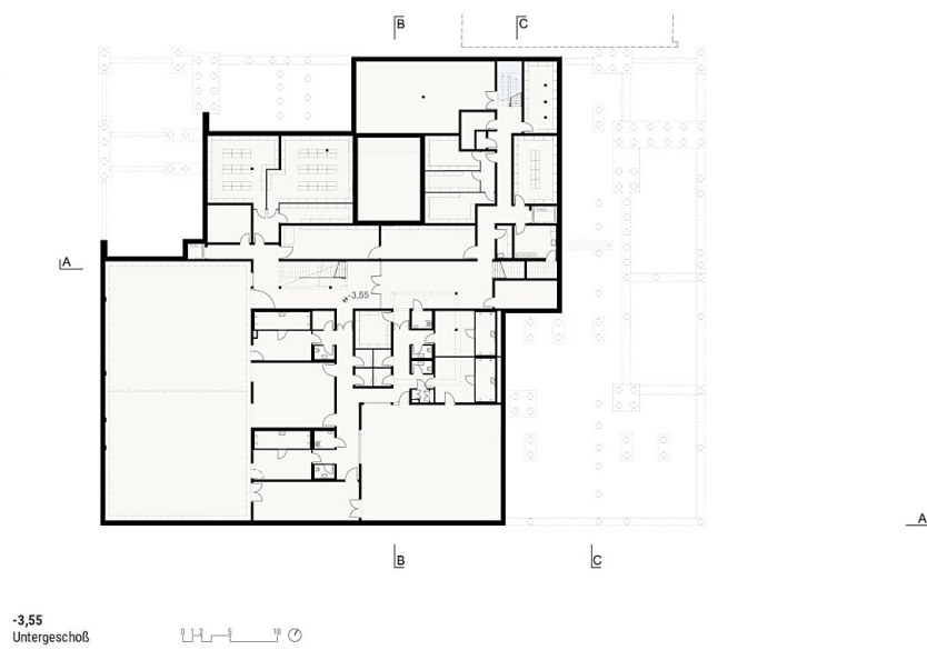
Grundriss UG1
