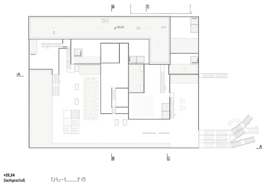
Grundriss DG
