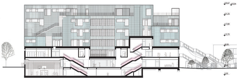
Cluster - Raumaufteilung
