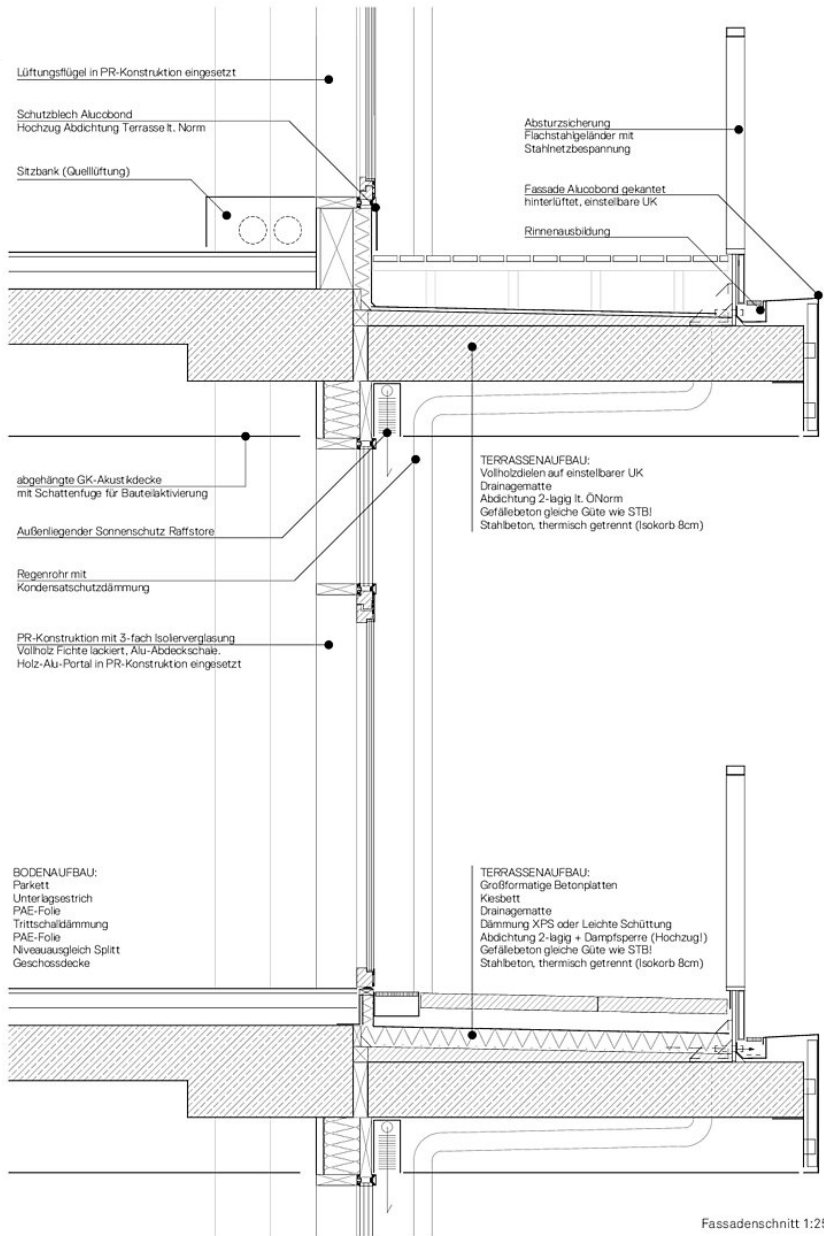
Fassadenschnitt
