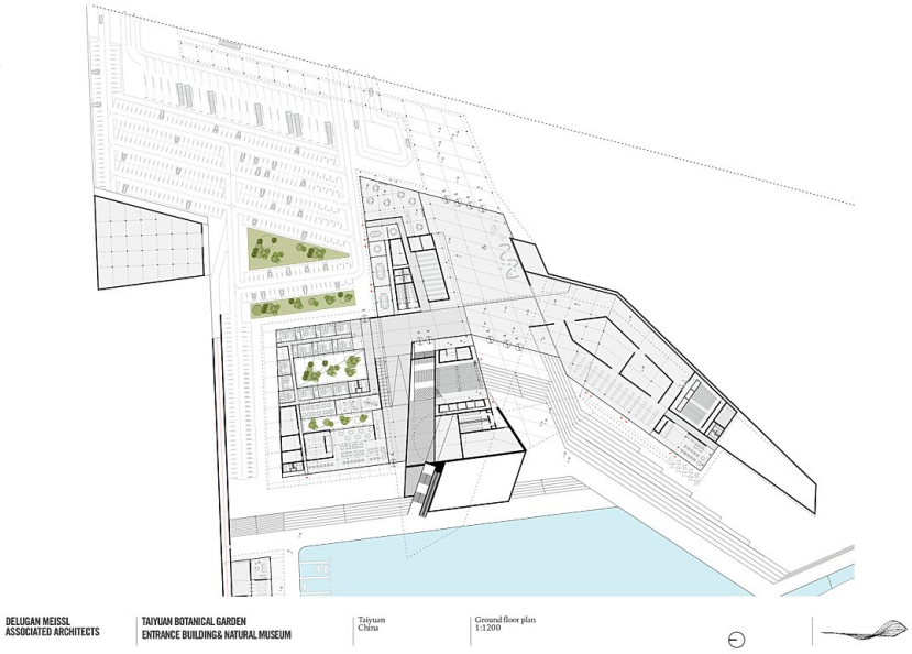
Grundriss Museum EG
