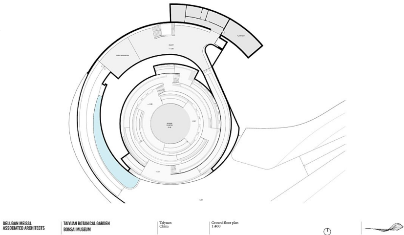
Grundriss Bonsai Museum EG
