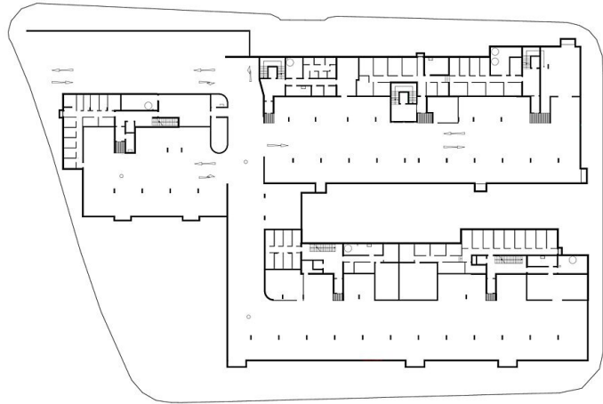
Untergeschoss 1:500
