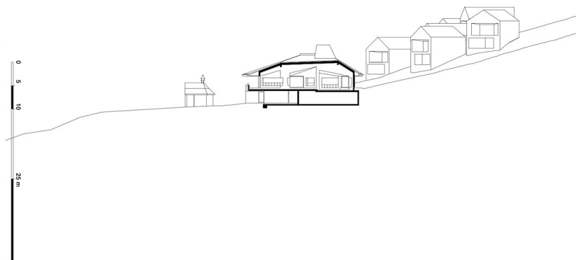
Schnitt (Haupthaus)
