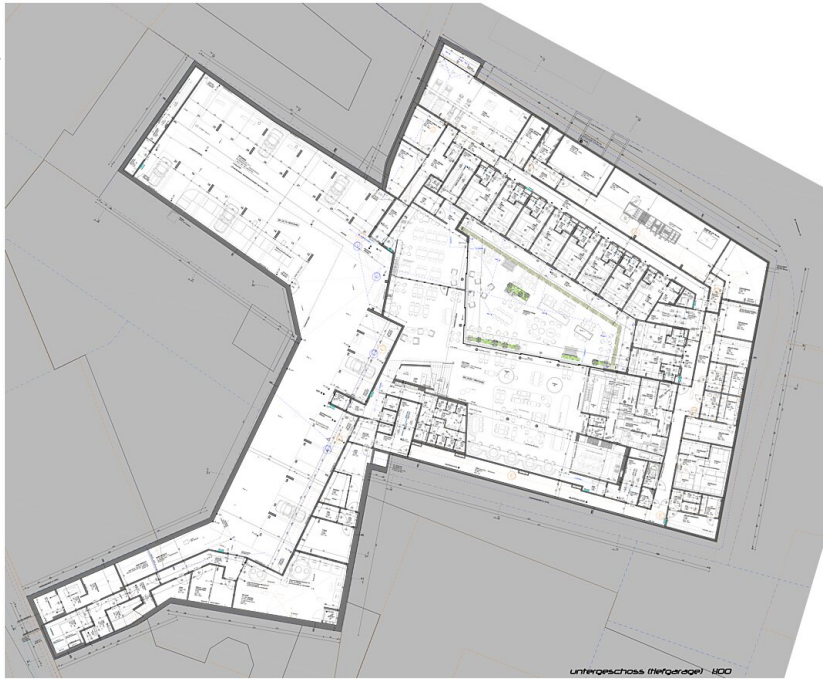
Grundriss UG
