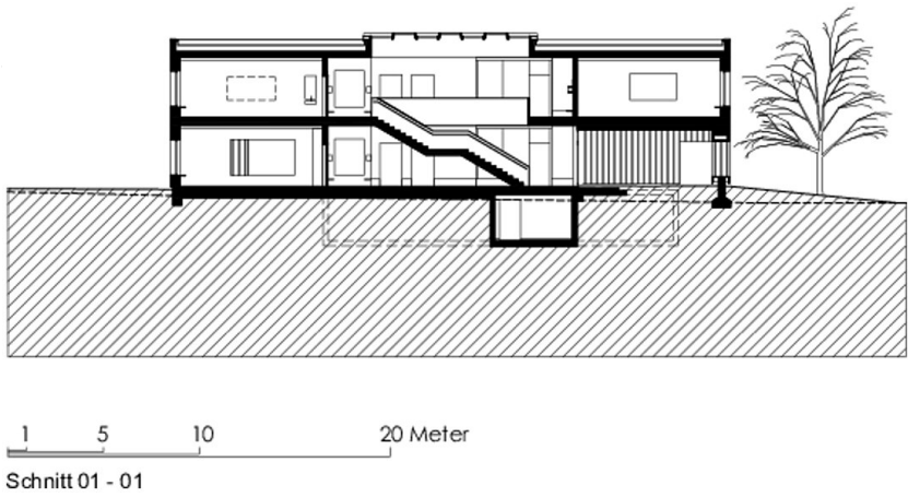
Schnitt
