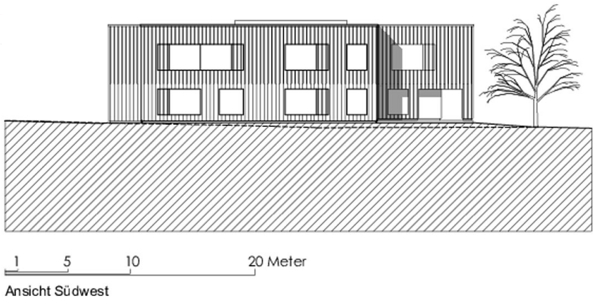
Ansicht SW
