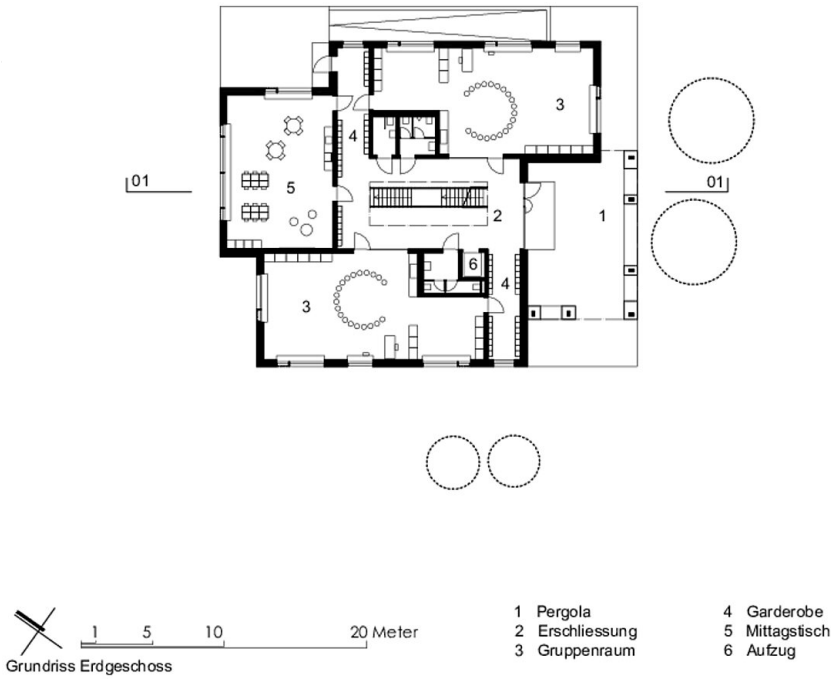
Grundriss EG
