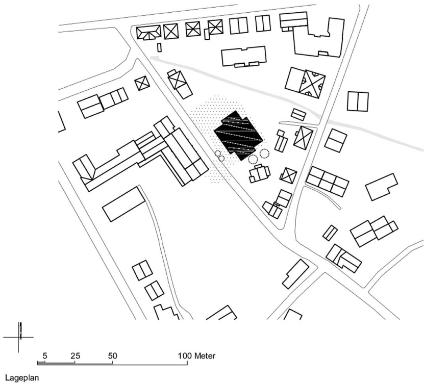
Lageplan
