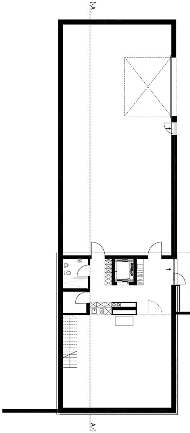
Grundriss EG
