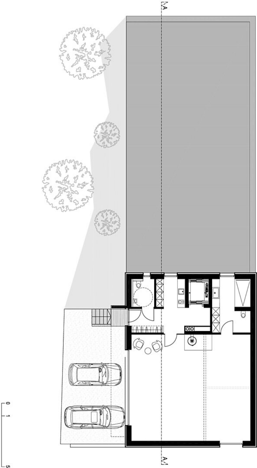
Grundriss OG
