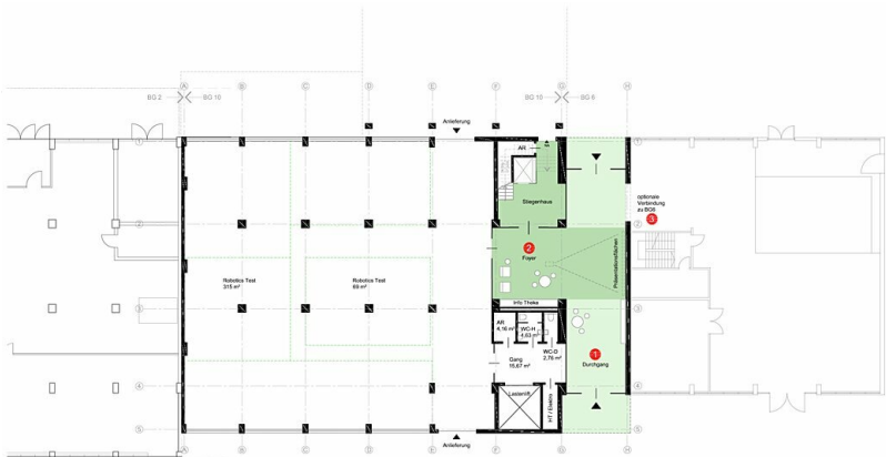
Grundriss Erdgeschoss M 1:200 1. frei bleibender Durchgang (optional: Infoboard) 2. Zentraler Foyerbereich; übersichtliche Zugangssituation; nutzbar zur Firmenpräsentation 3. mögliche Verbindung ins BG6
