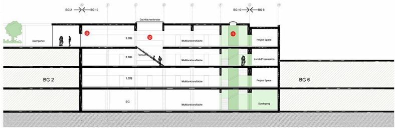
Schnitt M 1:200 1. Farbkonzept, Signalfunktion - Wegesystem / Orientierungsbeschriftung 2. Verbindungstreppe im Bereich Mittelzone als zentrales, natürlich belichtetes Verbindungselement 3. optionale Anbindung - Belebung Dachgarten
