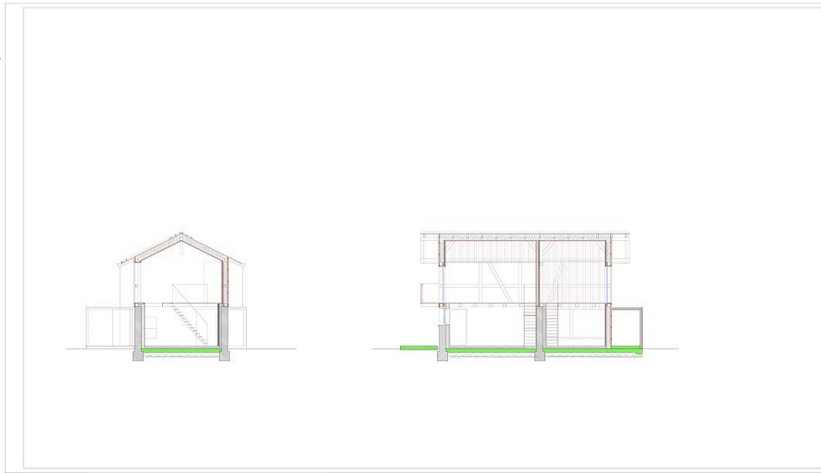
Schnitte
