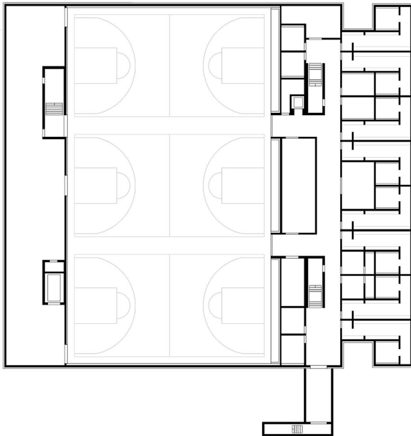
Grundriss E1
