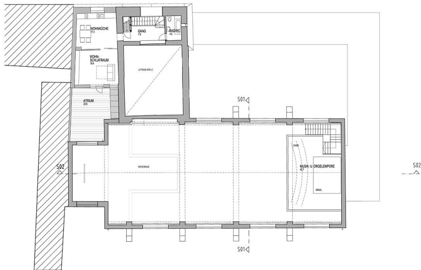
Grundriss OG
