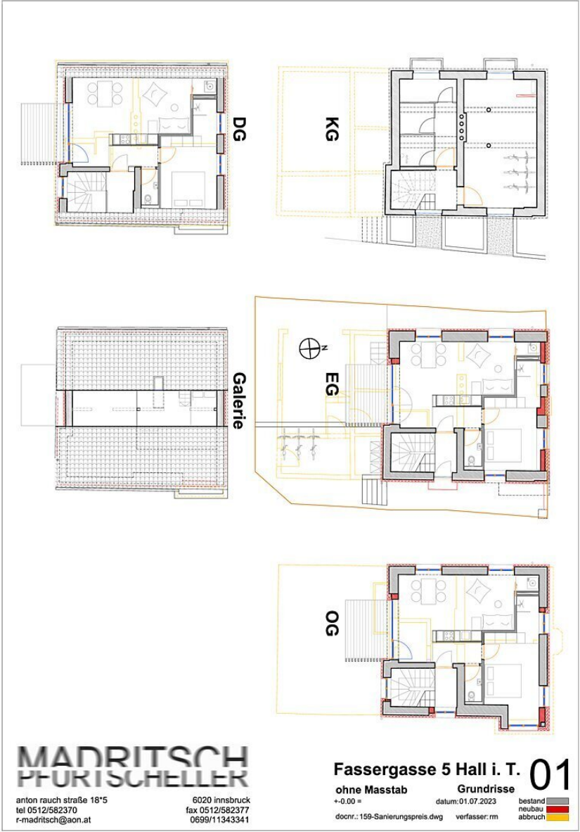
Grundrisse
