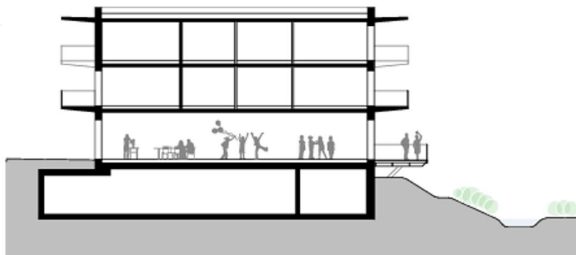
Schnitt B
