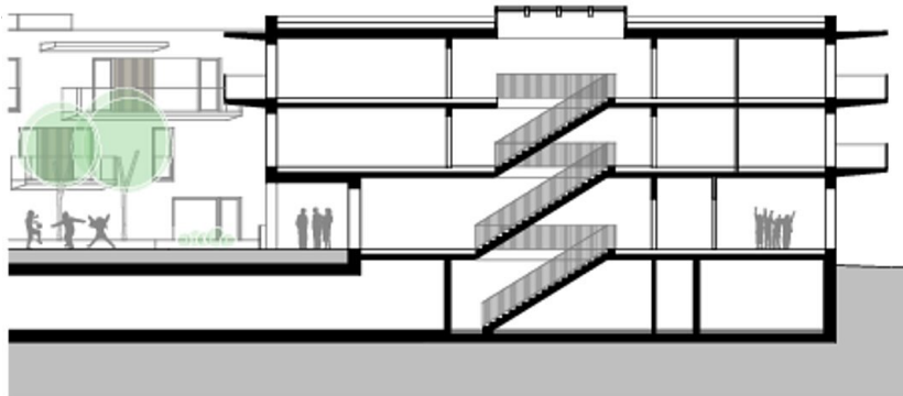
Schnitt A
