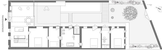
erdgeschoss M 1:100
