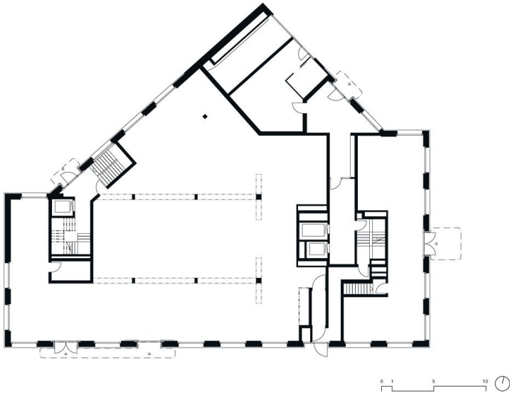
Grundriss EG
