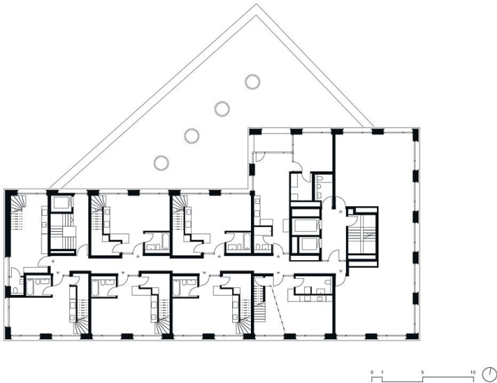
2. Obergeschoss
