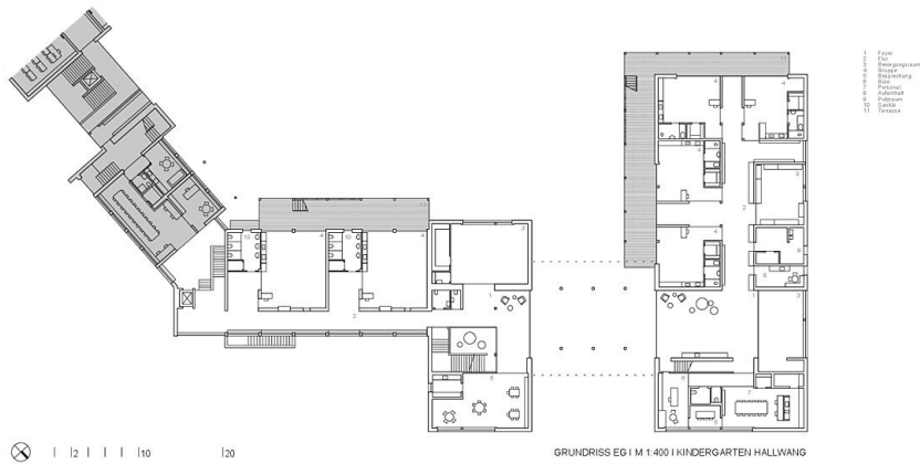
Grundriss EG
