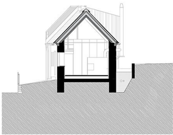
Schnitt B-B 0 1 5 10
