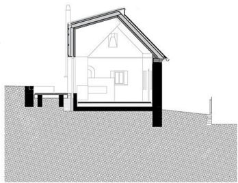
Schnitt D-D 0 1 5 10
