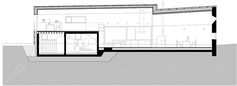
Schnitt A-A 0 1 5 10
