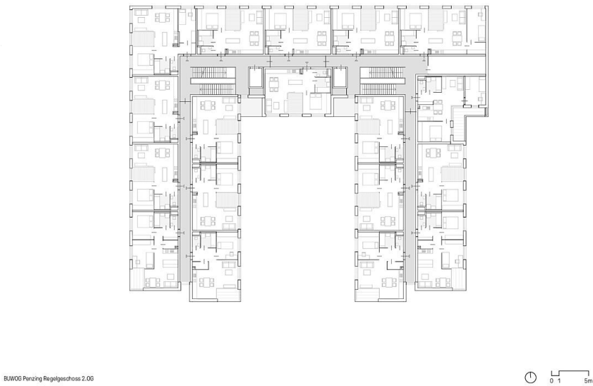
Grundriss RG
