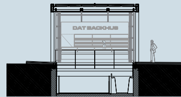
Querschnitt Backhaus M 1:250
