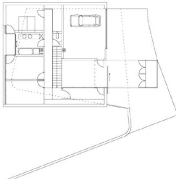
Grundriss
