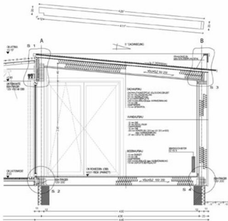
GESAMTSCHNITT 1 - 1
