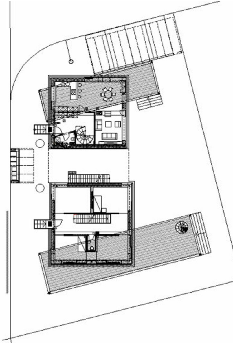
Grundriss OG
