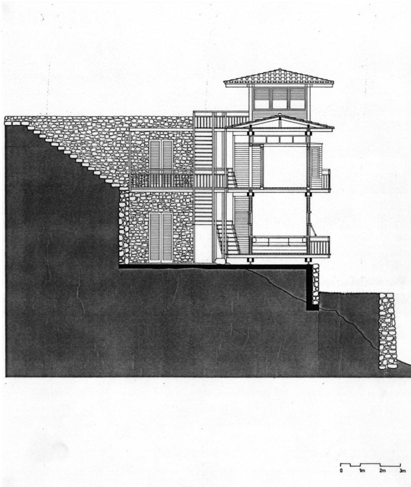
Querschnitt
