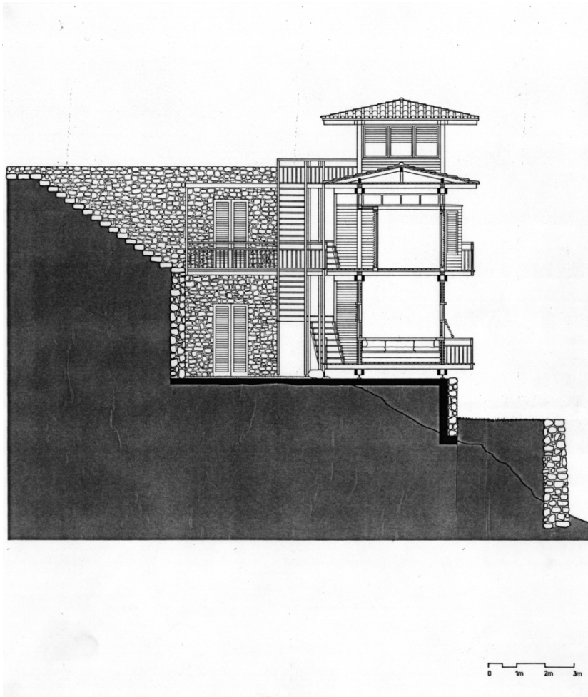
Querschnitt
