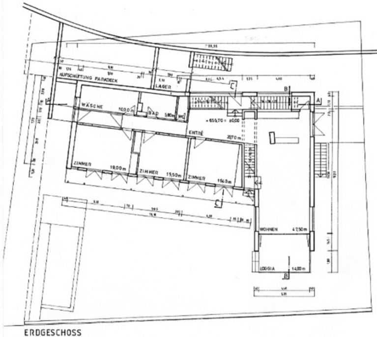
ERDGESCHOSS
