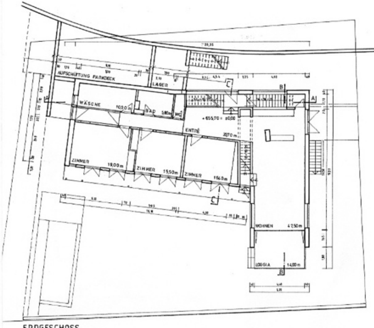
ERDGESCHOSS
