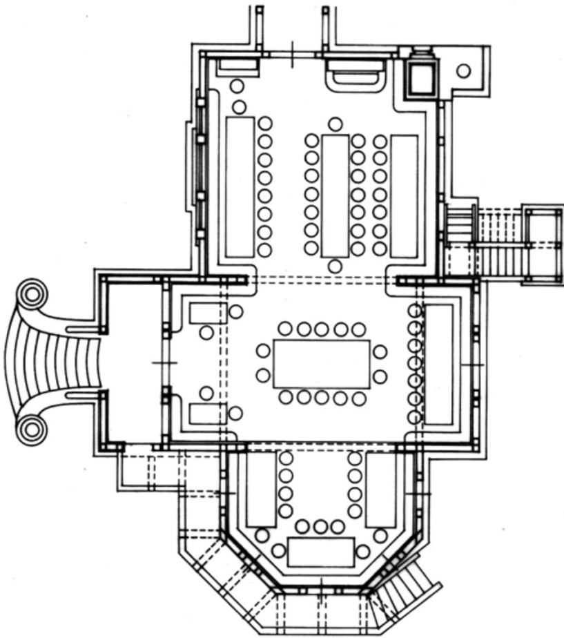
Grundriss
