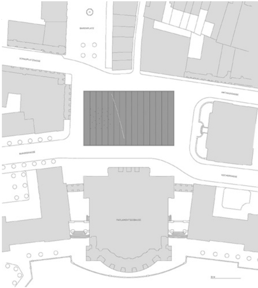
Lageplan
