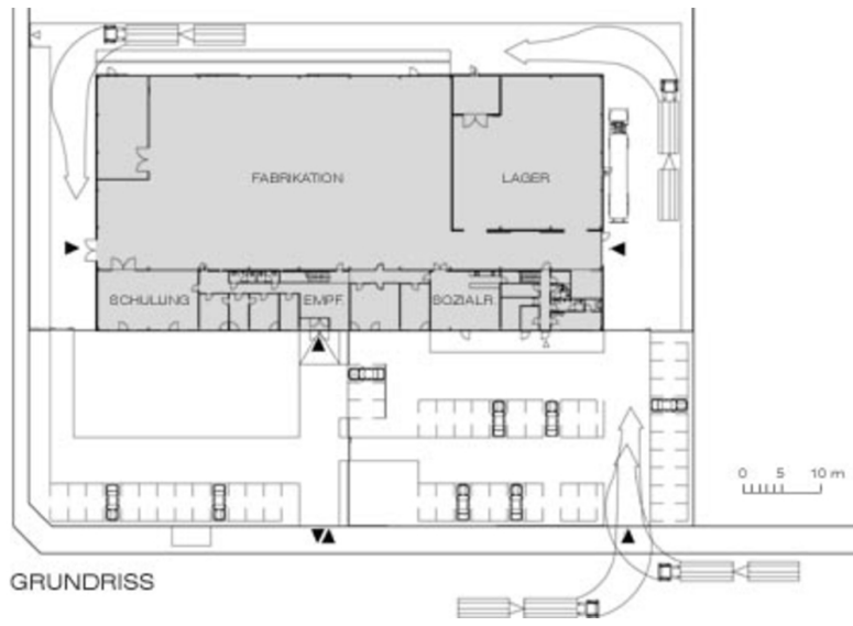
Grundriss
