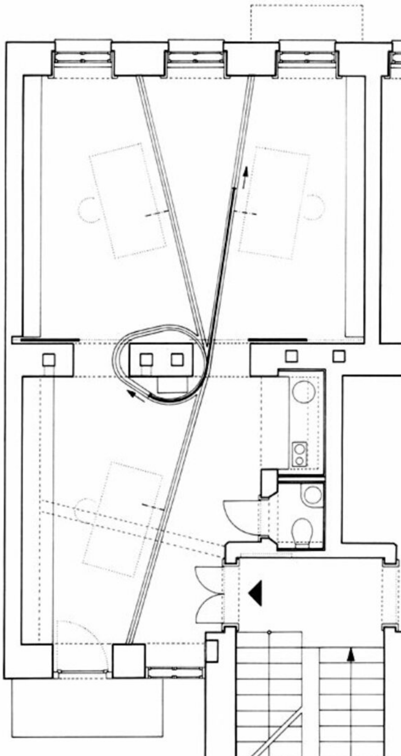
Grundriss
