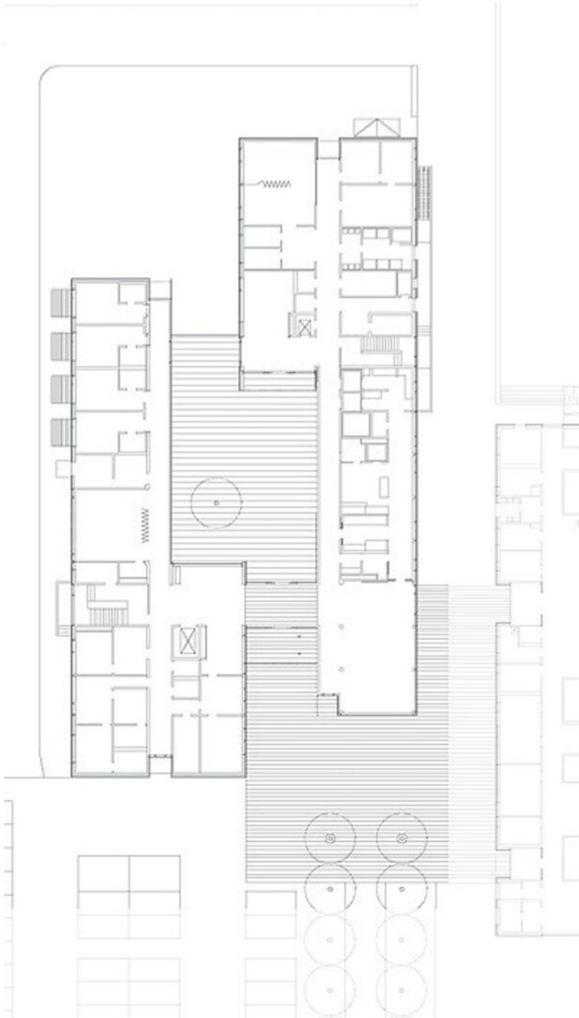
Grundriss EG
