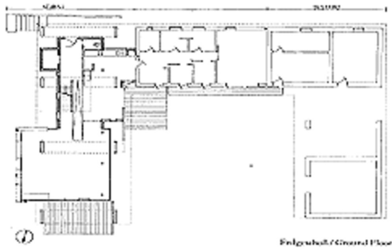
Grundriss EG
