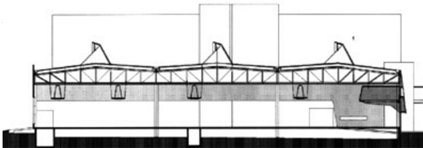
Schnitt Produktionstrakt
