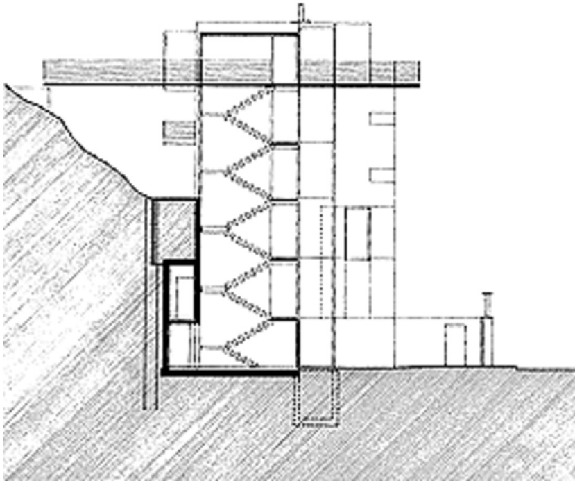
Schnitt
