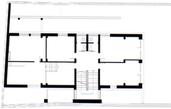
Pôdorys 1. PP
