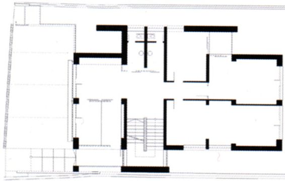
Pôdorys 1. NP
