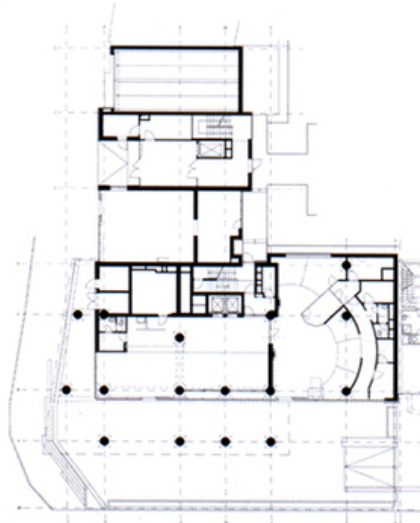
Pödorys 1. NP
