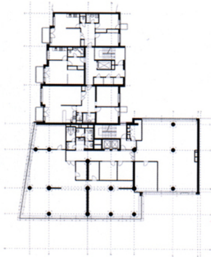
Pödorys 6. NP
