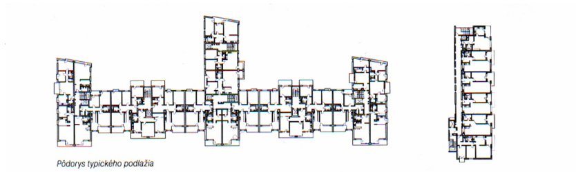
Pôdorys typického podlažia
