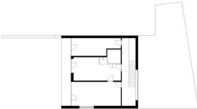
GRUNDRISS OBERGESCHOSS
