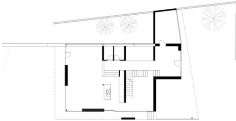
GRUNDRISS ERDGESCHOSS
