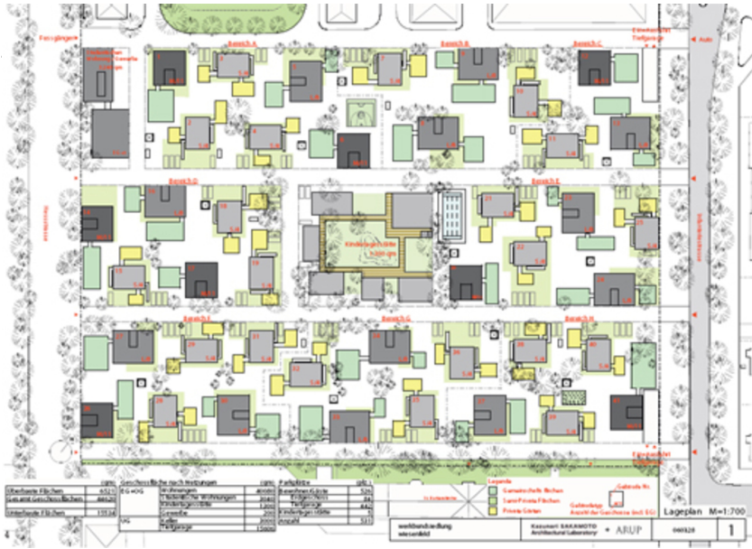
Lageplan
