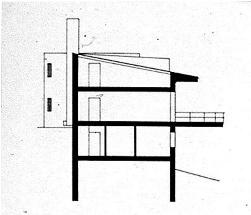
Querschnitt
