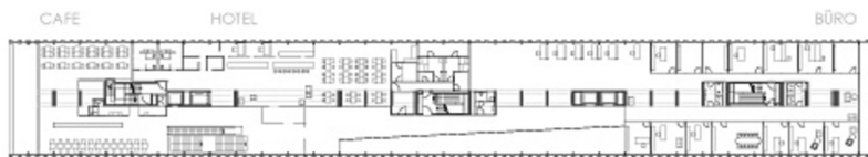
obergeschoss 1 m 1:500
