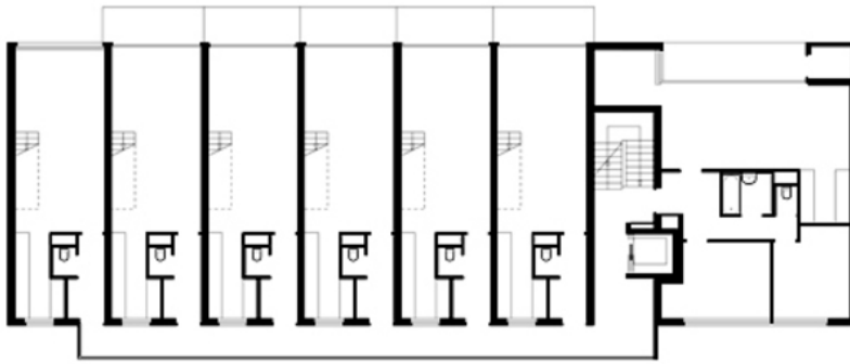
GRUNDRISS 2./4. STOCK
