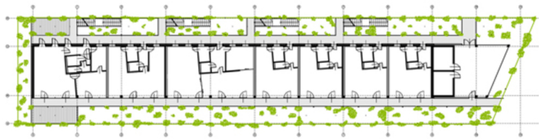
Grundriss EG
