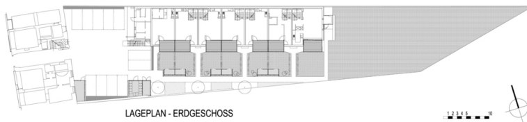
LAGEPLAN - ERDGESCHOSS
